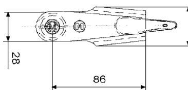
Lanový závěs pro lanko OR 6mm
